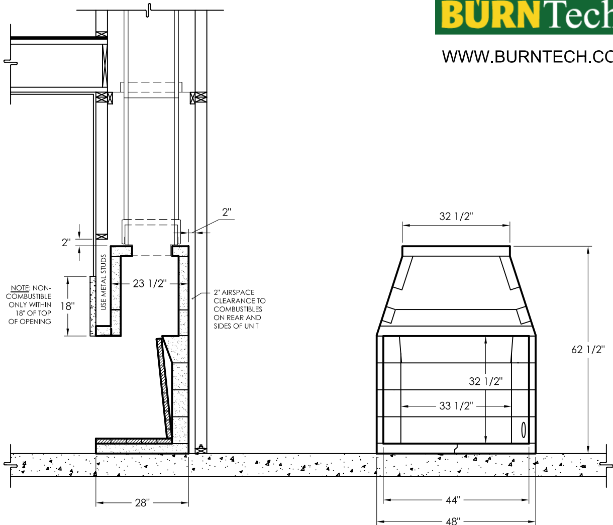
SECTION A-A
